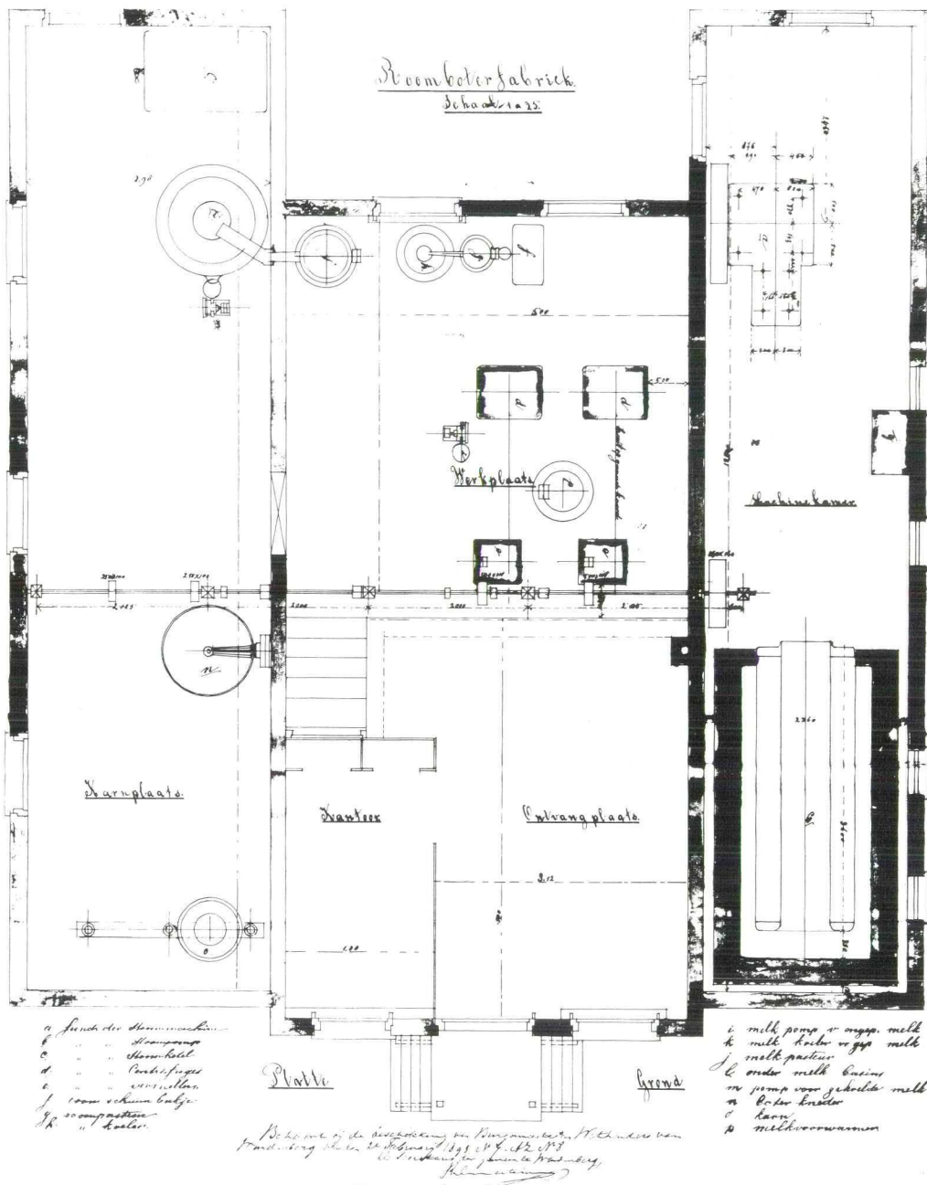
Plattegrond Stoombooterfabriek 'De Vooruitgang' van de uitbreiding in 1898. Ingericht voor het gebruik van een stoommachine.
