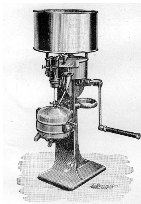
Melotte Handcentrifuge
