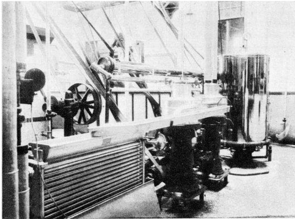
5. . . . in de „pasteur“, als consumptiemelk (de ketel rechts op de foto) of in de beide daarnaast opgestelde centrifuges, die de room en de ondermelk scheiden; de room wordt afgekoeld door de geheel links staande geribde koeler.
