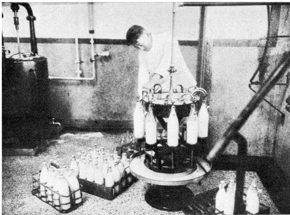
7 De automatische vuling der melkflesschen.
