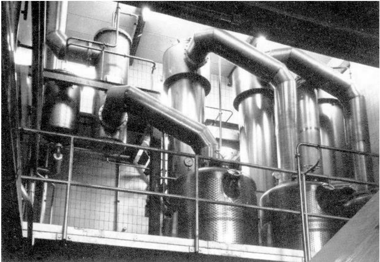
Indampinstallatie
