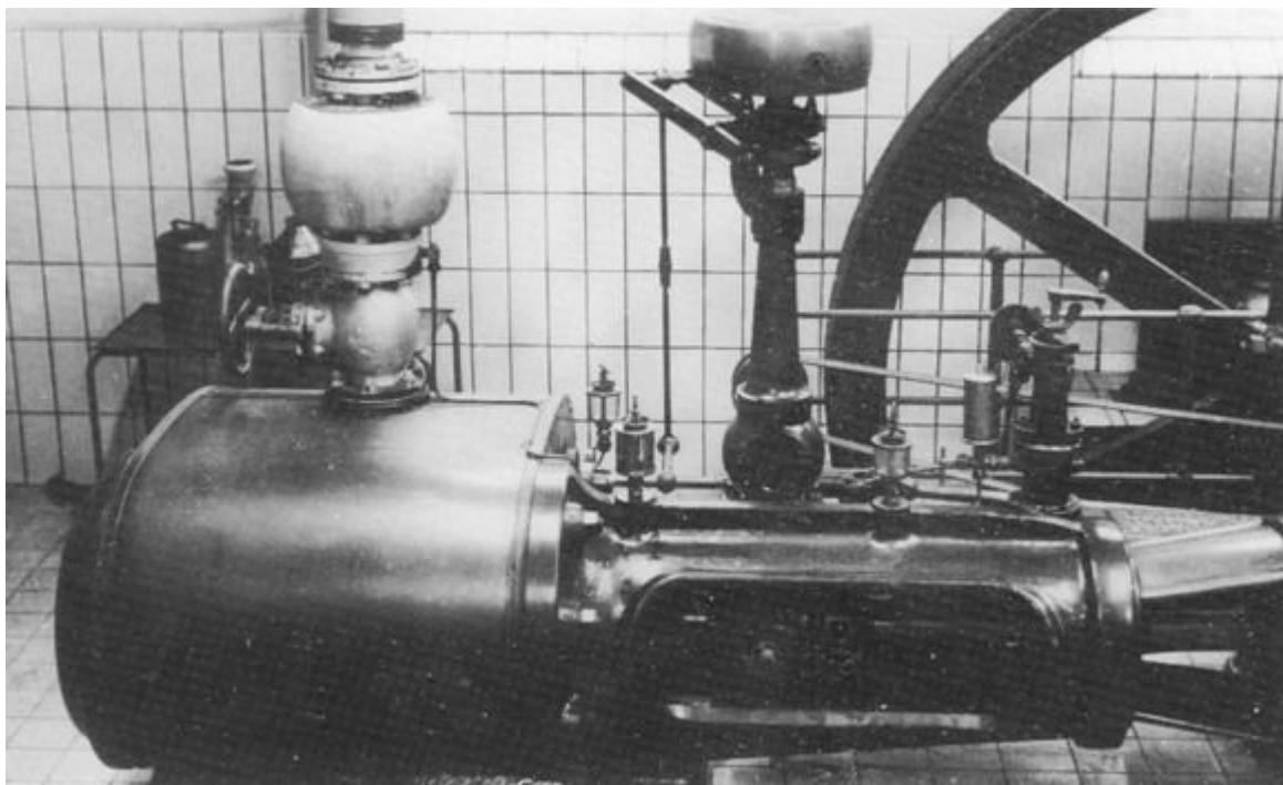
Zestig pk stoommachine uit 1927 Veertig jaar later werkte deze nog.
