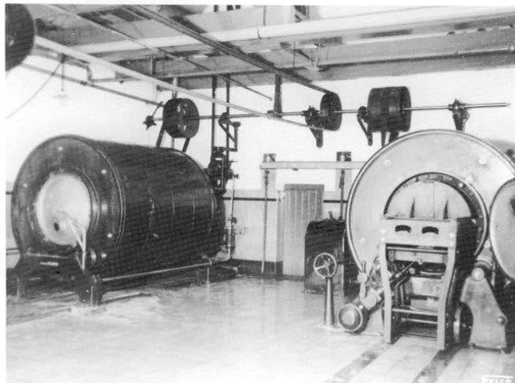
Een karnlokaal met de vóór de Tweede Wereldoorlog algemeen gebruikte karnen
