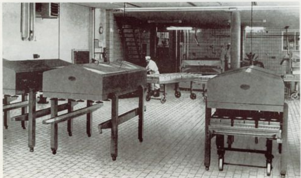
Pneumatische tafelpersen
