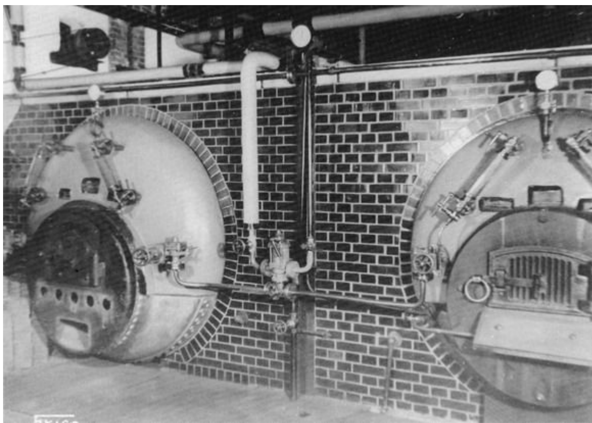
Een ketelhuis met, zoals dat vroeger gebruikelijk was, ingemetselde stoomketels.
