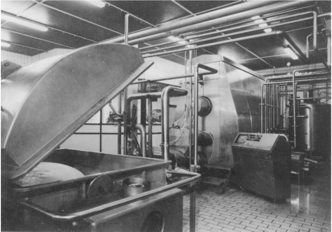
De botermakerij met een capaciteit van 5.000 kg boter per uur.
