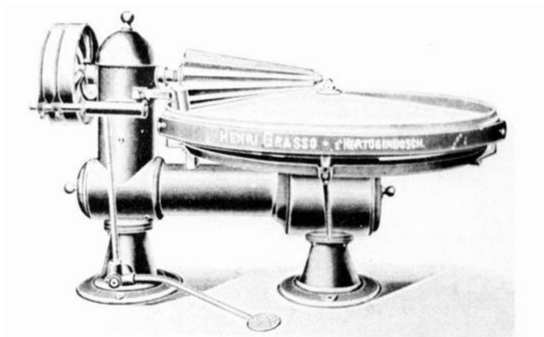
Een riemgedreven boterkneder, waarmee het water werd uitgekneed en de boter homogeen van structuur werd gemaakt. Met het voetpedaal kon de riemschijf in de vrijloop gezet worden.
