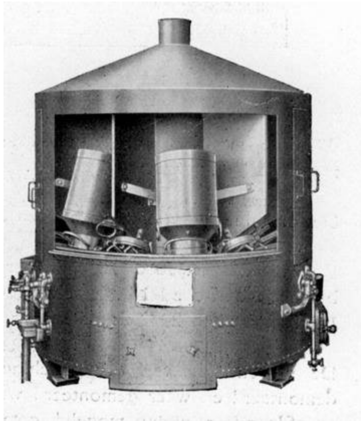
Kannenwasmachine rond model (foto zuiveljaarboek 1935)
