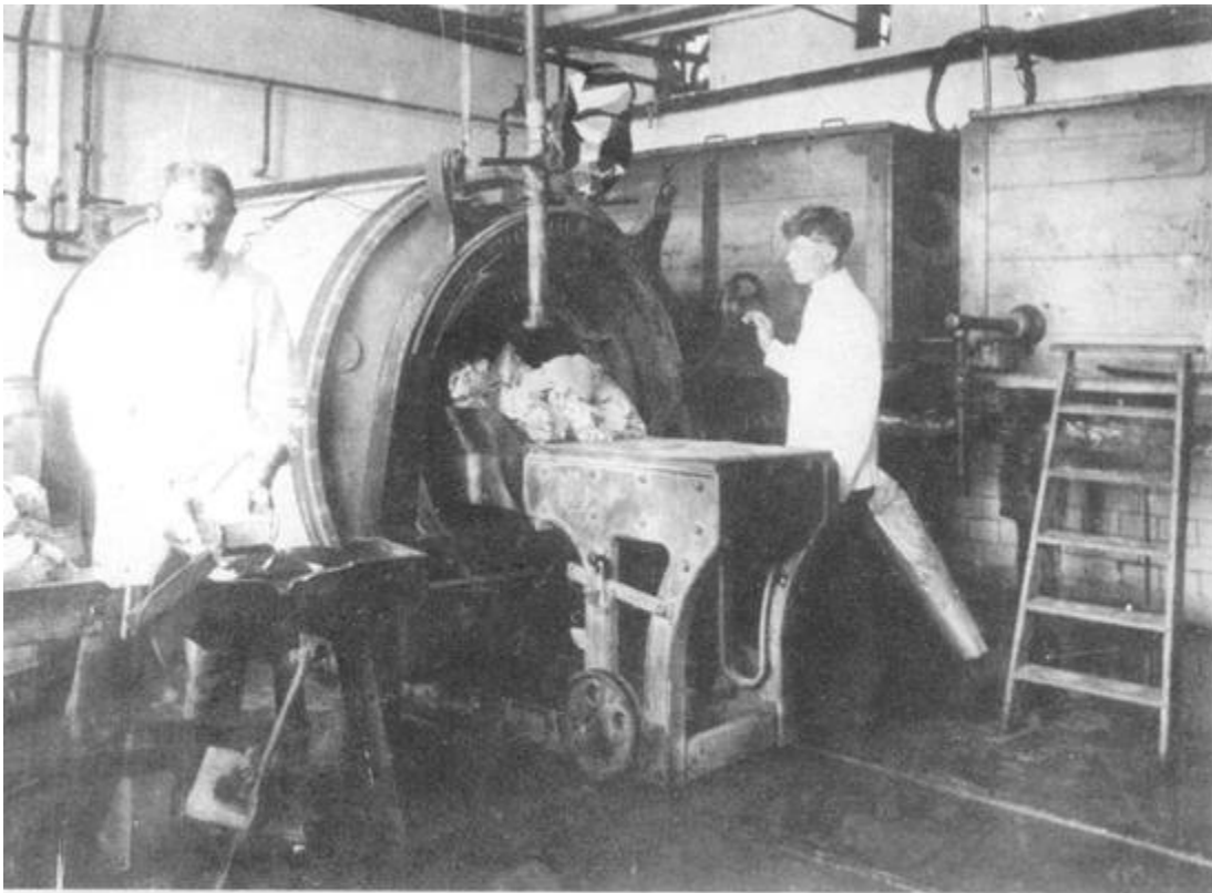
Een karnkneder met ingeschoven kneedwagen (foto "St. Martinus", Princenhage)
