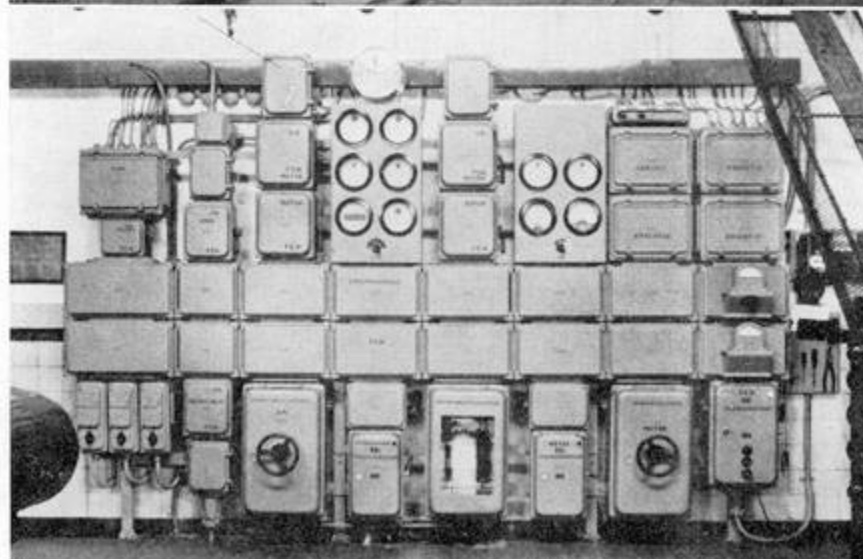
Schakelkast
