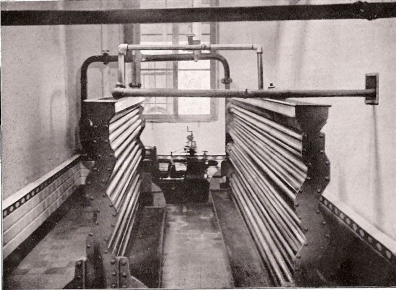
Koelerlokaal.
