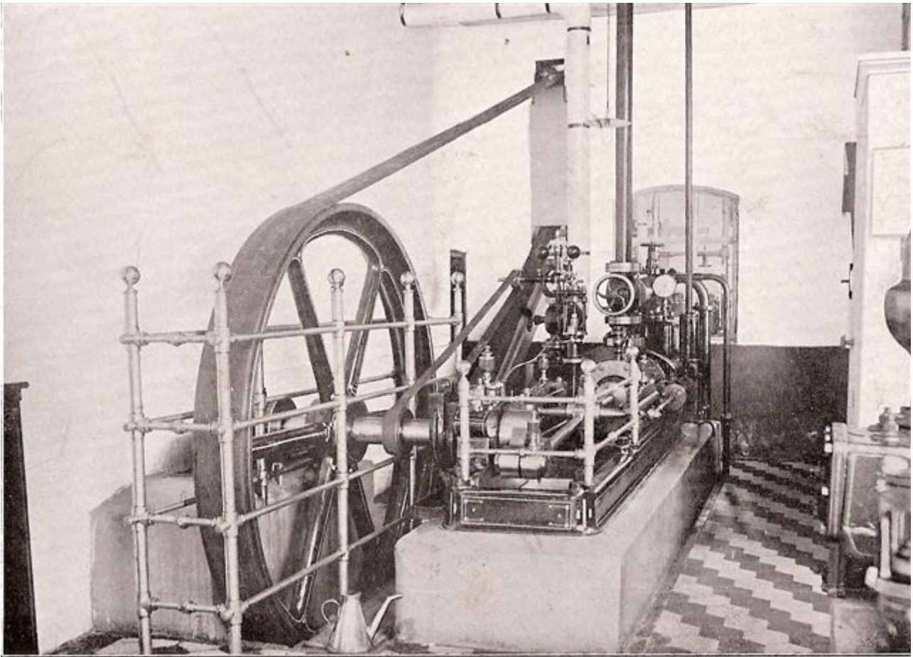
Machinekamer.
