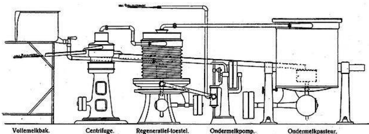
Fig. 74. Schematische voorstelling van de opstelling van de werktuigen in het centrifugelokaal van een boterfabriek.
