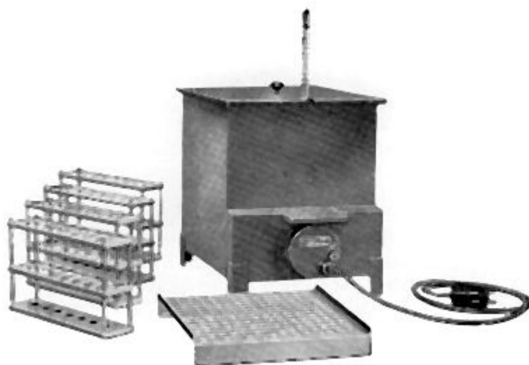
Fig. 32. Zelfreguleerd elektrisch waterbad voor butyrometers.
