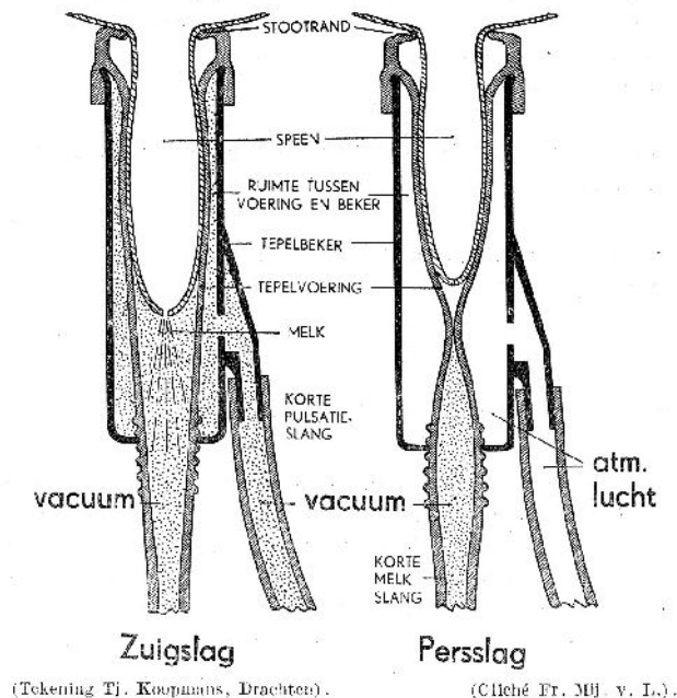
Fig. 9. De werking van de tepelhouder.
