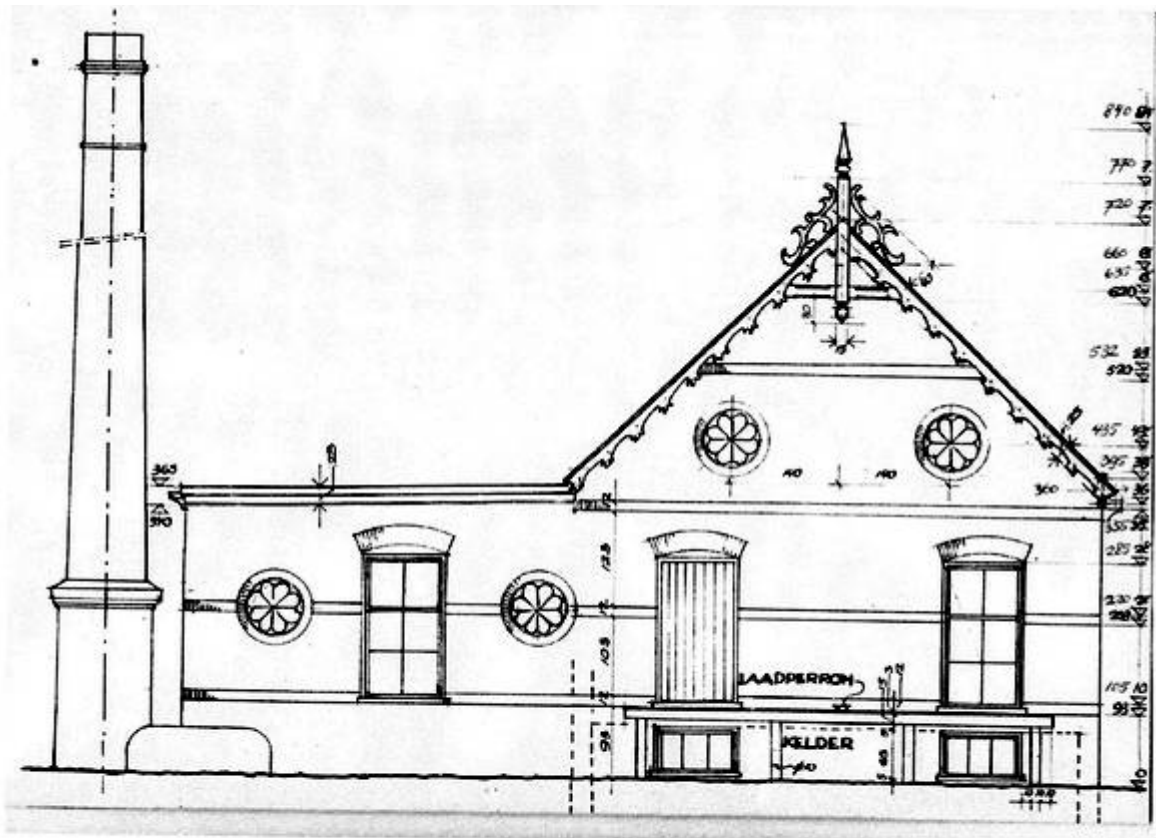
Gereconstrueerde bouwtekening van de uitbreiding van de 'Eensgezindheid'. Het gebouw met het puntdak (rechts) dat in 1900 is gebouwd, wordt in 1906 uitgebreid met een ruimte voor stoomketel en stoommachine en een schoorsteen. De stoommachine staat in de aanbouw links, achter het ronde raampje. (Met dank aan de heer B.K. Pater)
